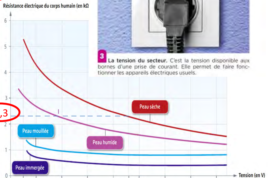
5 Résistance électrique du corps humain et tension de contact. Le corps humain est un conducteur de courant électrique. Le corps humain n'est pas un dipôle ohmique. On peut appliquer la loi d'Ohm au corps humain uniquement pour une valeur de tension fixée ou d'intensité fixée.
